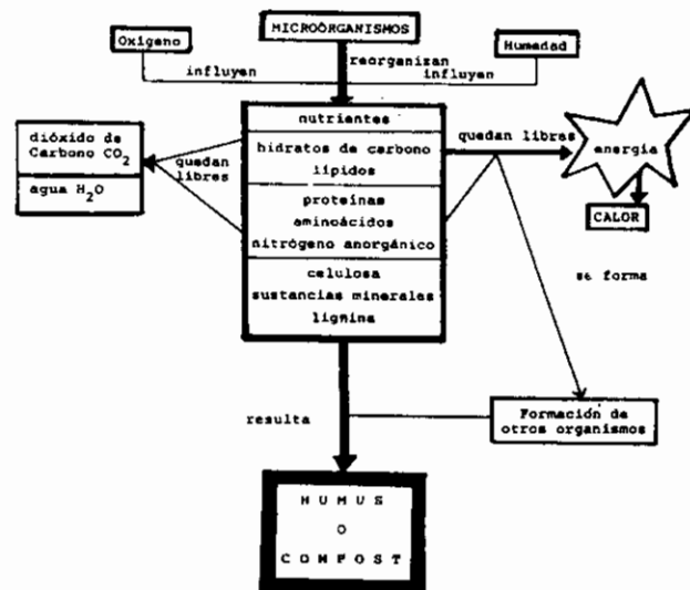
El proceso de transformación durante la descomposición de la materia orgánica en el compost (Fuente: Brechelt, A. 1996)
